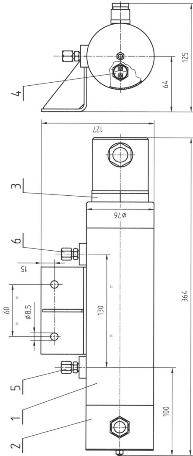
GO-0,6 Schița constructivă
